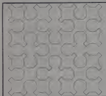
Figure 3. Sierpinski order 2.
